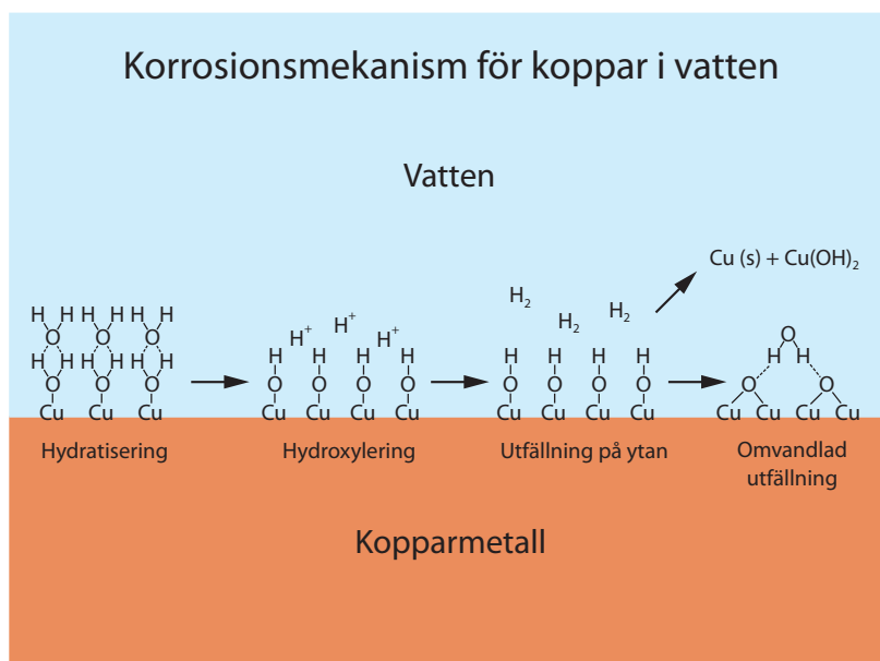
Figur 2 Översikt av en möjlig mekanism för korrosion av koppar i rent syrgasfritt vatten
